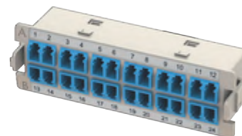
LC/UPC OS2 Module
